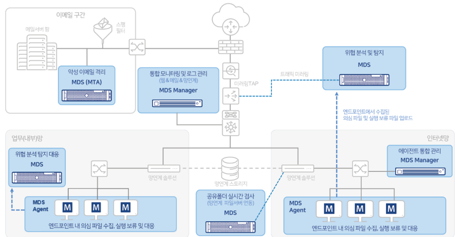
[그림 1] AhnLab MDS 구축 구성도
