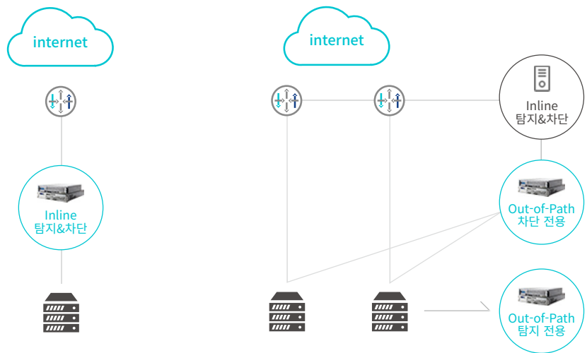
[그림 1] Inline vs Out-of-Path 구성 방식
